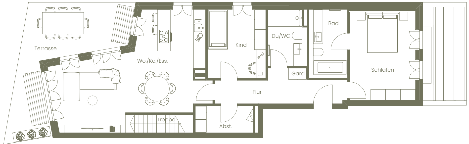
GARTENGESCHOSS
